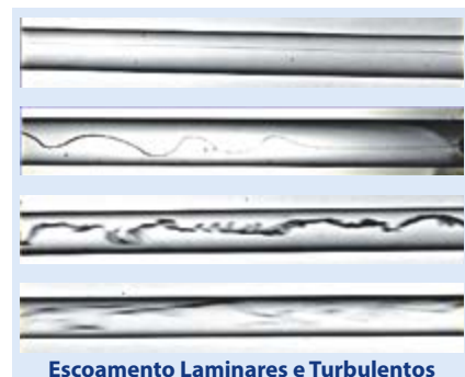
Escoamento Laminares e Turbulentos
