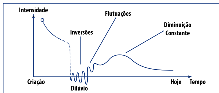
Figura 2: Variações do campo magnético da Terra
