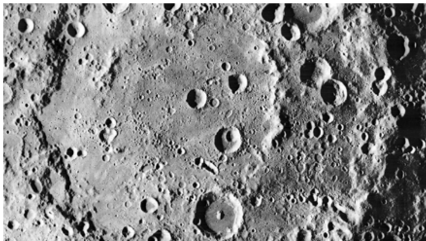
Crateras da Lua
