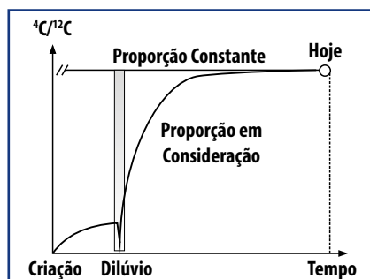
Figura 1: Alterações na proporção ^{14}\text{C}/^{12}\text{C} na atmosfera da Terra. 4
