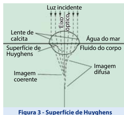
Figura 3 - Superfície de Huyghens
